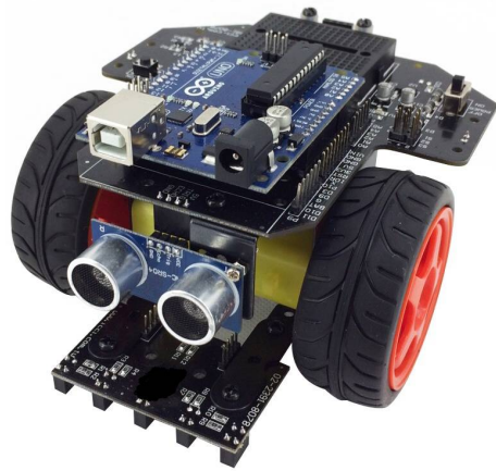
自走車循跡比賽參考作品
