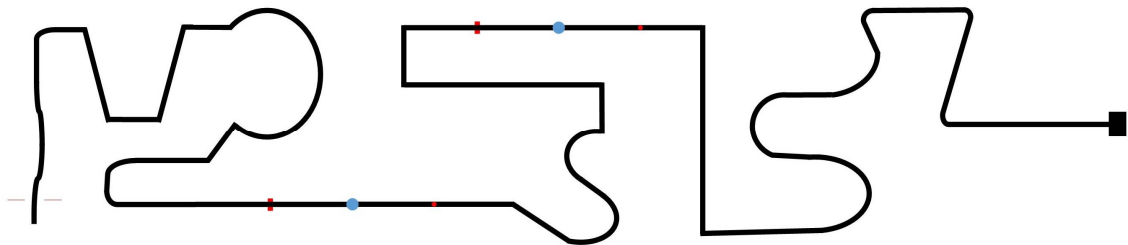
比賽場地圖(A) 尺寸:120 寬 x 480 長，單位:CM
